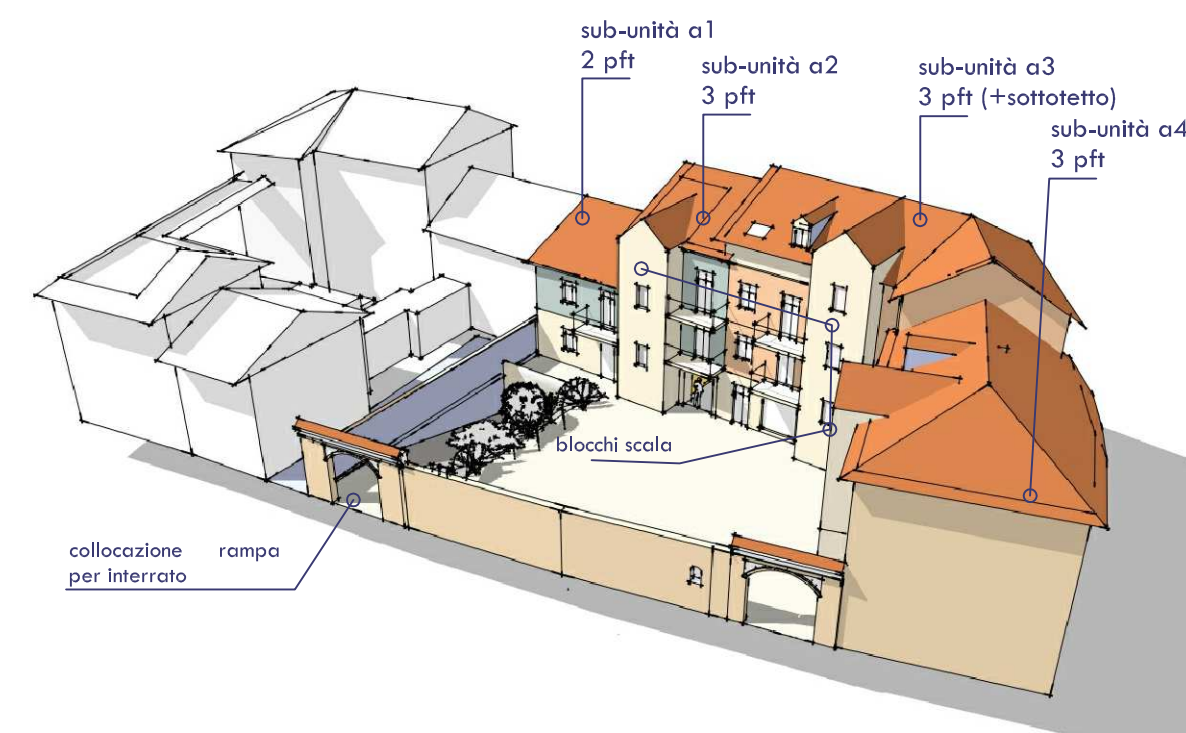
SCHEMA TRIDIMENSIONALE PROGETTO
